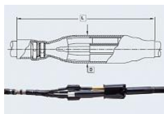
Переходная муфта TRAJ-12-1x150-400 (097)
