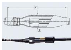
Переходная муфта TRAJ-12-1x70-120-CEE01 (097)
