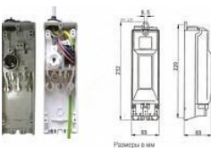
Соединительная коробка EKM-2020-1D1-1SA
