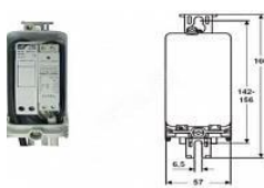
Соединительная коробка EKM 2045-1FNT-M
