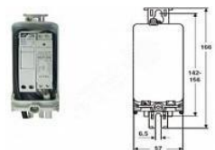
Соединительная коробка EKM 2045-1FNT-G
