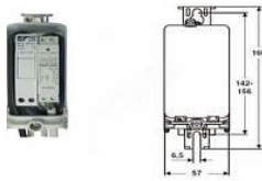
Соединительная коробка EKM 2045-1FN-M
