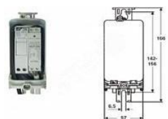
Соединительная коробка EKM-2050-2D1-5S6-U
