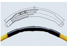
Ремонтная муфта REPJ-42-1x70-120
