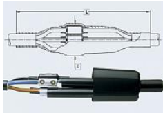
Комплект для оконцевания СИП SMOE 81976
