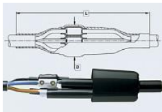
Соединительная муфта SMOE-81140
